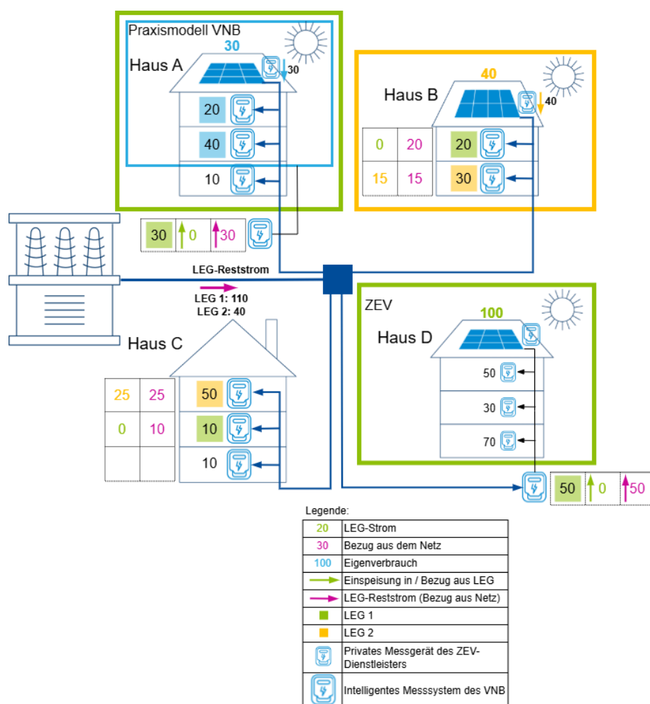
Abbildung 6 LEG mit Praxismodell VNB (in Bezugssituation) und ZEV
